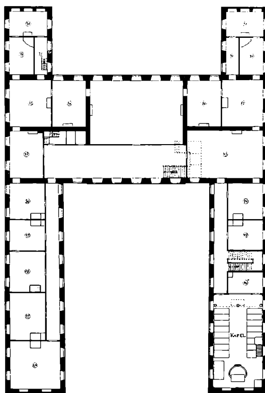
CLAUSCLA. PLAN AF 1 STE SAL.
