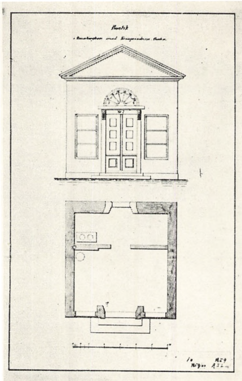
Murermester D. V. Kleins forslag fra 1859 til ombygning af pavillonerne i Kronprinsessegade.
