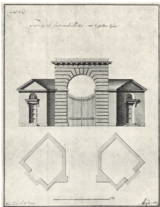
Tegning af Peter Meyn til Gothersgadeporten, forelagt Rentekammeret 1802 (Litra B. i P. Meyns skrivelse af 29. marts 1802). Mål: ca. 1:250.
