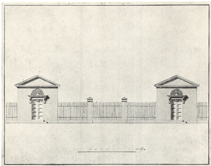
Samtidig kopi af Peter Meyns tegning til pavilloner for enden af Dronningens Tværgade, forelagt Rentekammeret 1802 (Litra C. i P. Meyns skrivelse af 29. marts 1802). Mål: ca. 1:250.
