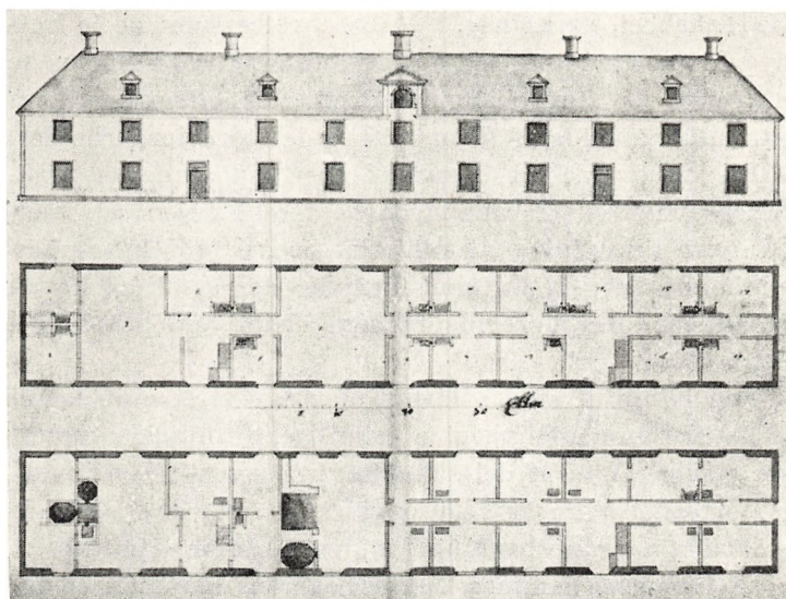
Vestfløjen på Hirschholm slot 1727. Tegningen skyldes vistnok J. C. Krieger. (Rigsark.).
