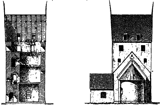
SNIT AF TAARNET FRA S-N.
