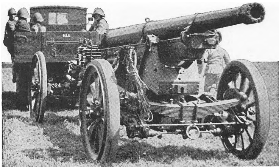
TUNG 10,5 CM KANON I KØRESTILLING
