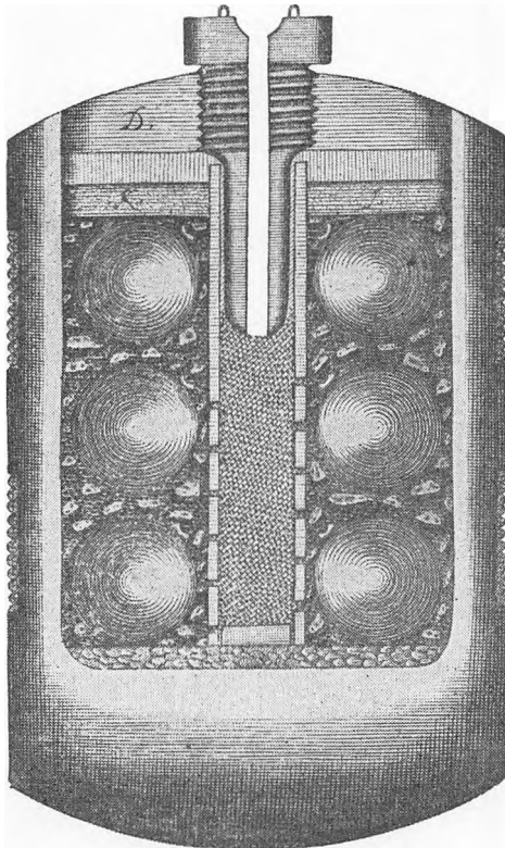
60-PUNDIG BRANDGRANATKARDÆSK FRA DET 17. OG 18. AARHUNDREDE
