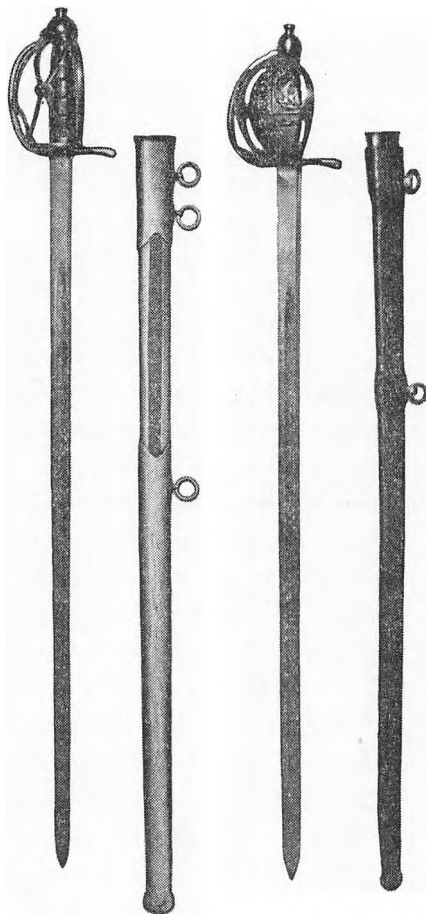
PALLASKER FRA FREDERIK VI.'s HÆR Findes paa Tøjhusmusæet. Fra venstre Rytterpallask Model 1789. Messingfæstet en Ændring fra Model 1774. Skeden af Jern, Model 1779: Pallask for Livgarden til Hest, Model 1808. Messingfæstet fra Dragonpallask 1785, monteret paa Klingen fra Rytterpallask 1789. Skede af brunt Læder. — Fot. Tøjhusmusæet.
