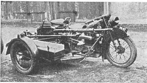
MOTORCYKLE MED PAAPRODSET 20 MM KANON Kanonføreren, den tappert kæmpende Sergent Løvgrens, Maskine efter Kampen ved Bredevad, den 9. April 1940. Fot. Jessen.
