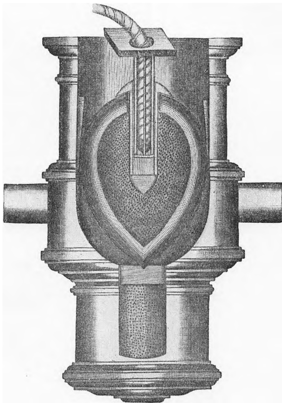
TVÆRSNIT AF HÆNGEMORTÉR FRA DET 17. OG 18. AARHUNDREDE
