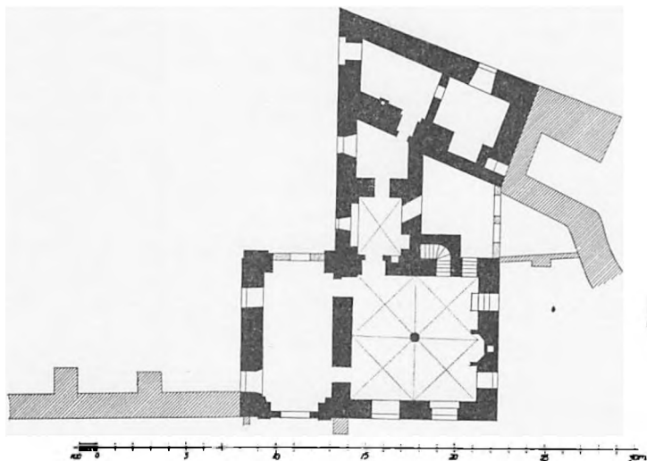
Fig. 86. Porthuset med endnu staaende Tilbygninger samt de i 1921 foretagne Udgravninger (de skraverede Partier). Efter Opmaaling af L. Thaysen og Kaj Uldall.
