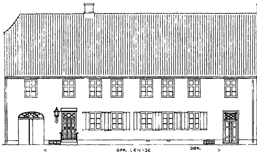
Lindegade 21, Apoteket. Facadeopmåling 1946.
