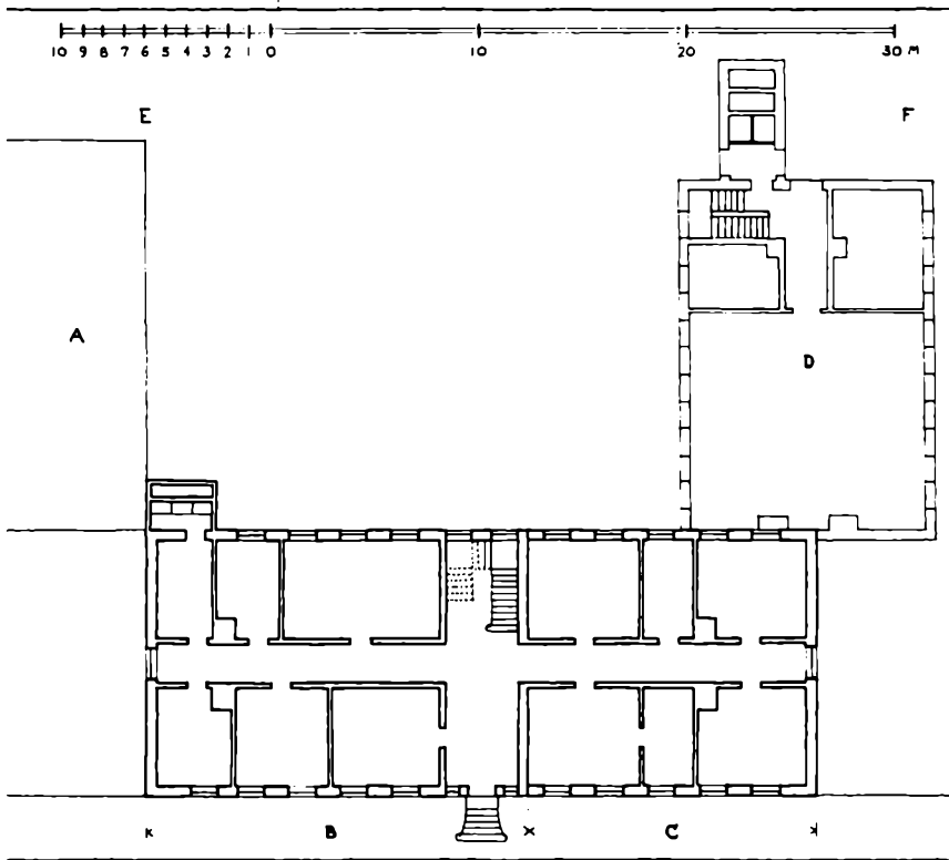
Søstrehusets plandisposition med midtergang og tværgående forstue. Bygningsanlægget i 1785 efter opførelsen af den østre sidesfløj. A. Vaskehus opført 1775, B. Vestre del af hovedbygning 1776. C. Østre del af hovedbygning 1780–81. D. Østfløj med korsal i 2. etage 1784–86. E. Vestfløj 1799–1800. F. Forlængelse af østfløj 1798–99. Rekonstruktion gengivet i mål 1:400. HHE (AB).
