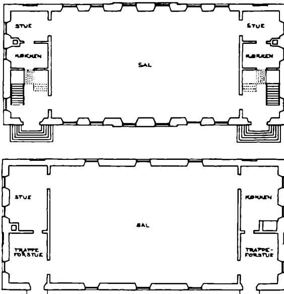
Planer i 1:400 til salshuset. Øverst planen fra 1775. Nederste plan er udtegnet på grundlag af Unitetets skriftlige anvisninger.
