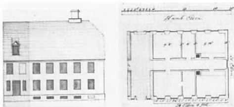
Udsnit (facade og stueplan) af bygningstegning til Søstrehusets østre del opført 1780–81. Tegningen indlagt i byggesagen Her gengivet i mål ca. 1:700.
