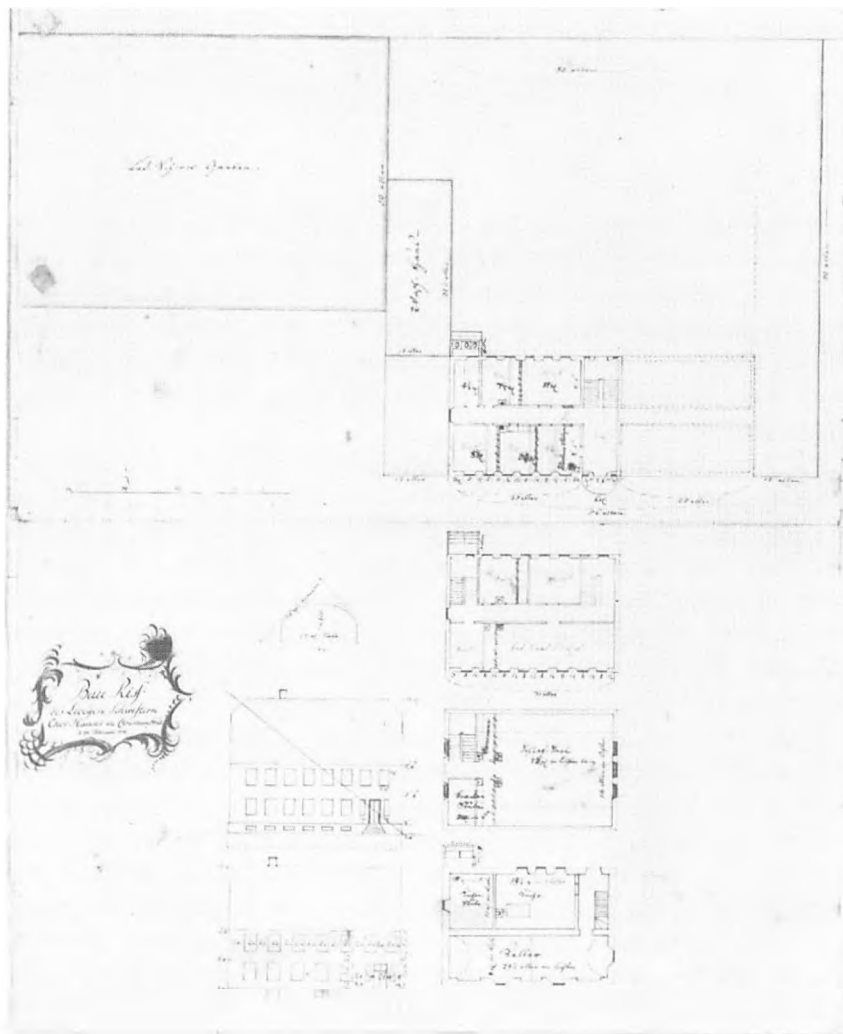
Bygningstegning til Søstrehusets vestre del dateret 22. februar 1776 (indheftet i byggesagen). Den foreslåede facade er streget ud og den udførte facade omfattende 7 vinduesakser (i stedet for 8) er tegnet nedenunder. Også på stueplanen er der foretaget rettelser. Gengivet i mål ca. 1:700.
