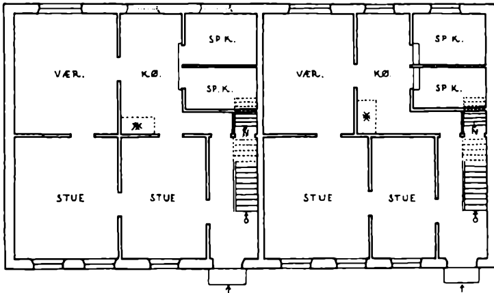
Lindegade 14–16 (V.kv. 15 og 14). Usymmetrisk dobbelthus opført 1794 af murermester Chr. Herzer, som beboede den østre halvdel. Plan og facade i mål 1:200 tegnet af HHE (AB) på grundlag af de arkitektstuderendes opmåling fra 1946.
