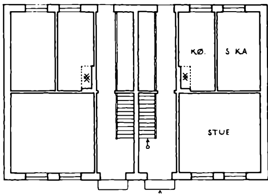
Lindegade 30-32 (Ø.kv. 1 og 2). Byens første dobbelthus opført 1774. Bemærk kvaderlisé- nerne på hjørnerne. Nørregade 3 B (Ø.kv. 20) opført 1780. Rekonstruktionsforsøg i mål 1:200 udført af HHE på grundlag af beskrivelse og bygningsundersøgelse. (AB).
