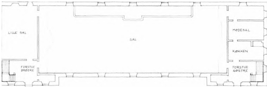
Plan i 1:400 af salshuset efter udvidelsen i 1796-97.
