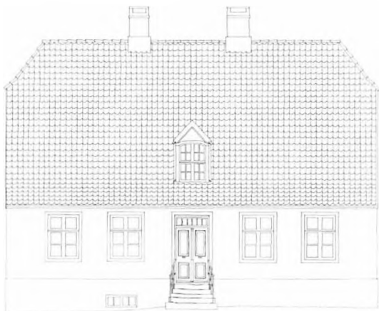
Nørregade 7 (Ø.kv. 18). Symmetrisk tofamiliehus. Plan tegnet af AB på grundlag af opmåling foretaget i 1946 af studerende på Kunstakademiets Arkitektskole. Facade reproduceret direkte efter opmålingen. Mål 1:200.
