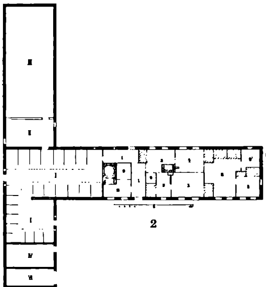
Fig. 2: Bondegård på Rømø. Jævnf. Fig. 3. I Stald, II Lo, III Lade, IV Faaresti, VI Vognskjul. 1 Fremgulve, 2 Køkken, 3 Sønnerdørns, 4 Nørredørns, 5 Kamre, 6 Pisel, 9 Bod, 9' Kælder, 10 Baggers.
