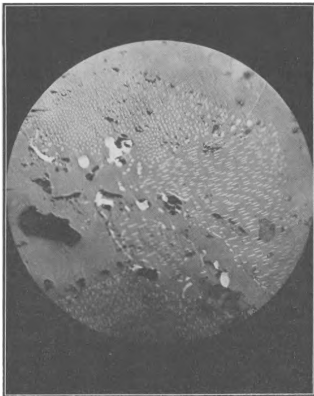
Mikrofotografier af Slaggeprøver, 125 Gange forstørret
