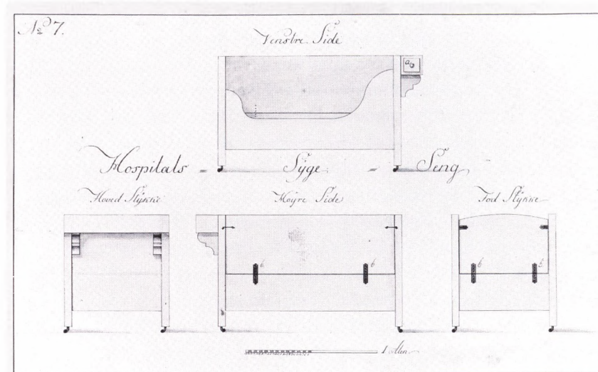
Tegning af sygeseng til »sygeindretningen« på Gråbrødre Hospital – fra 1790erne (V. Sylvest Frederiksen fot., Landsarkivet).
