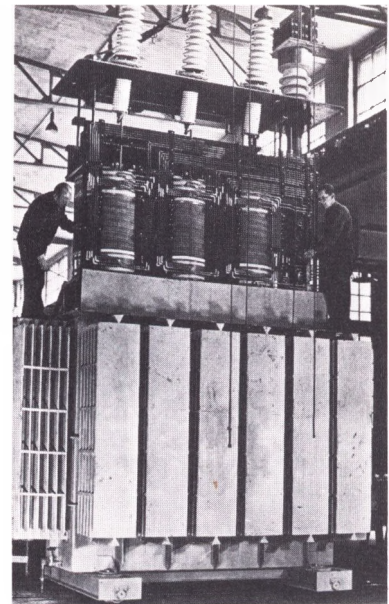
En transformator monteres hos Thrige.
