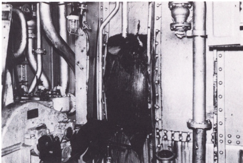
Hullet i skibssiden på »Linz« efter sabotagen den 28. juli 1943. (Rigspolitiets tekniske afdeling fot., Frihedsmuseet).
