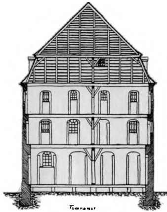
Tværsnit af Pakhuset.
