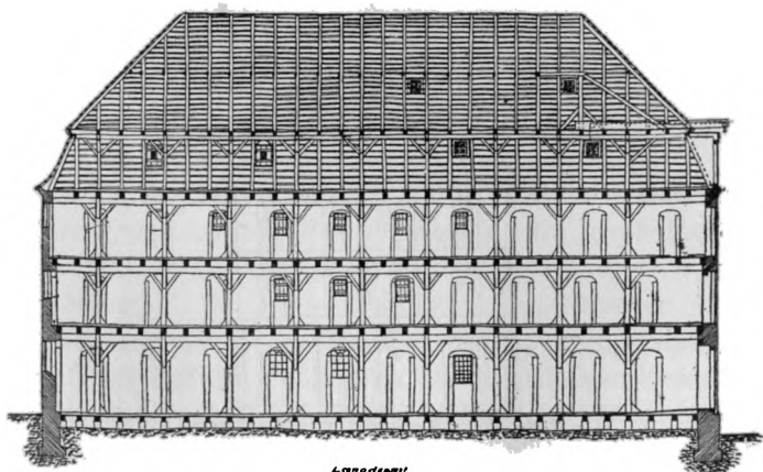
Længdesnit Længdesnit af Pakhuset.
