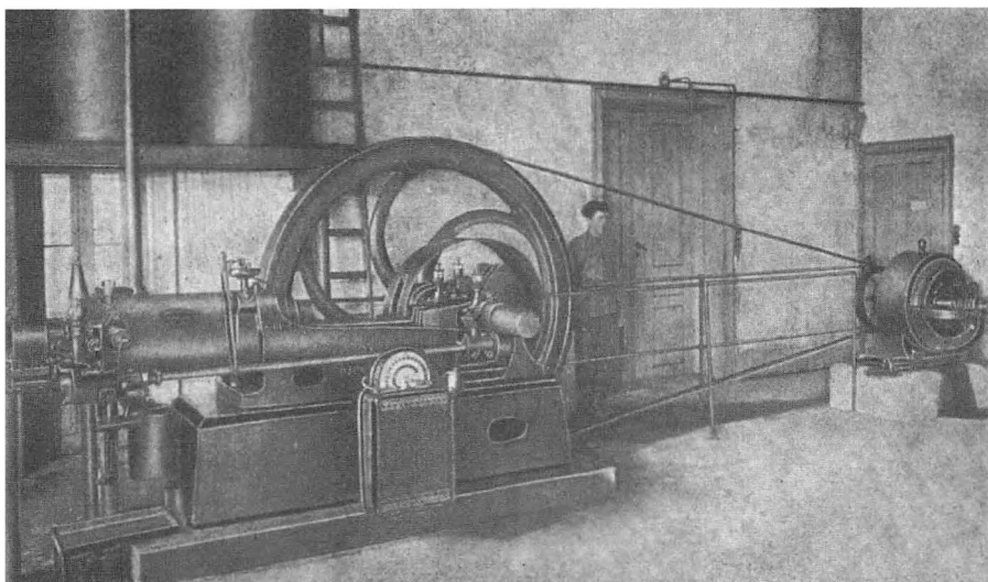
Fra et lille Elektricitetsværk – Gasmaskine og Dynamo.
