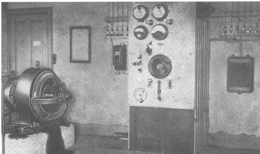
Fra et lille Elektricitetsværk – Dynamo og Fordelingstavle.
