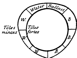
Tværsnit af Narval.
