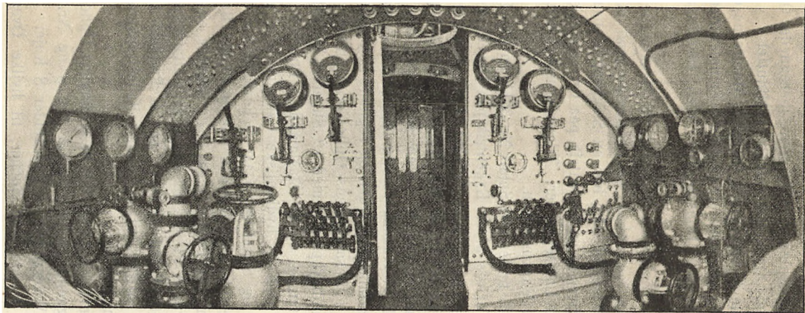
»Forkant af Maskinrummet med Strømfordelingstavle og Tilgangsventiler til Ballasttankene. Maalerne angive Vandstanden i Tankene. Gjennem Døren ser man ind i Kabyssen, fra hvilken et Mandehul fører op i Taarnet.»
