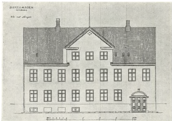
Opmåling af bispegården inden ombygningen i 1896. Side mod Nørregade.
