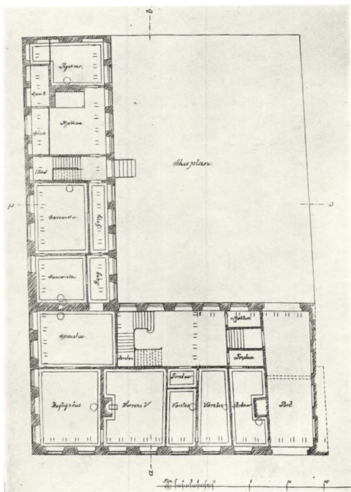
Stueplan af bispegården. Opmåling inden ombygningen i 1896.
