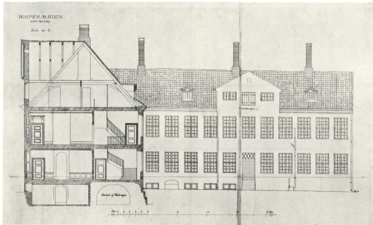
Opmåling af bispegården inden ombygningen i 1896. Snit og facade mod gården.
