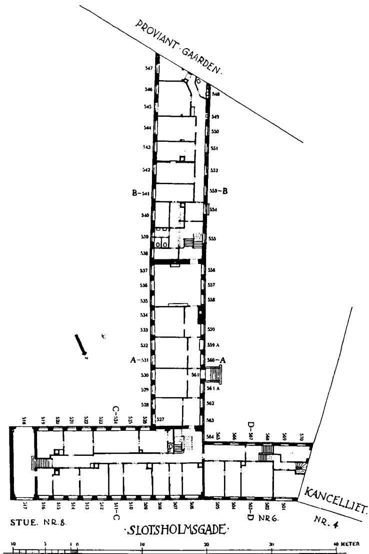
Slotsholmsgade nr. 8, tidligere Anna Sophie Reventlows palæ, plan af stueetagen. Slotsforvaltningen.
