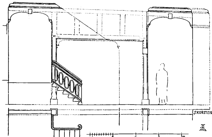
Rester af det oprindelige posthus i nr. 8, søjlerum, efter forfatterens opmåling.
