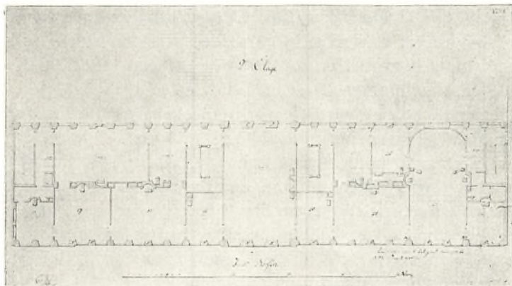
Slotsholmsgade nr. 10, oprindelig plan af 1. sal. Nationalmuseet.
