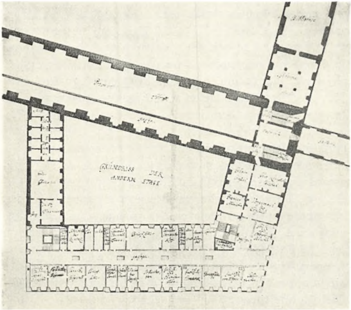
Kancellibygningen, plan af 2. etage. Rigsarkivet.
