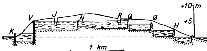
Fig. 8. Længdesnit af graven mod Sjælland
