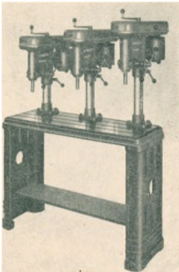
Hurtiggaaende Produktions-Boremaskine B.B.K. 13-3-M.A.
