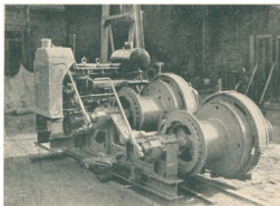
C.B.H. Rambukkespil
