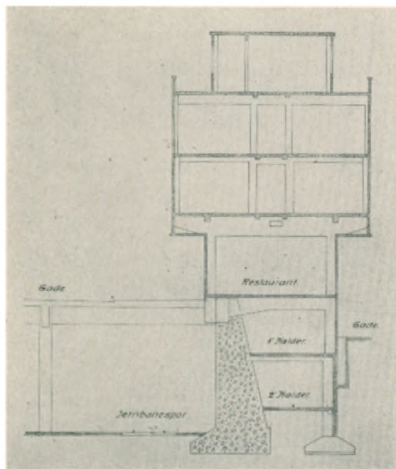
Hotel »Astoria« Tværsnit gennem Restauranten
