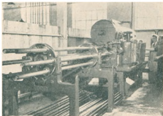
En af Firmaets moderne hurtiggaaende Maskiner
