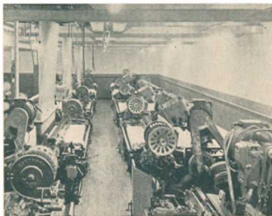
Moderne Vævehal med halvautomatiske Væve
