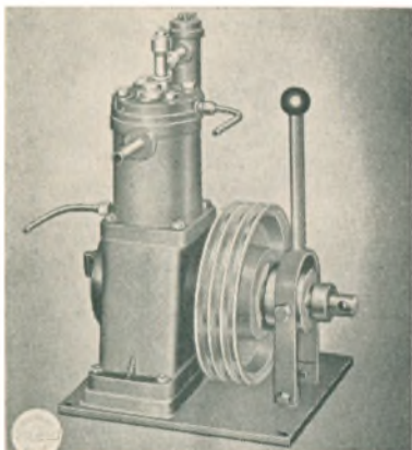
Startluftkompressor
