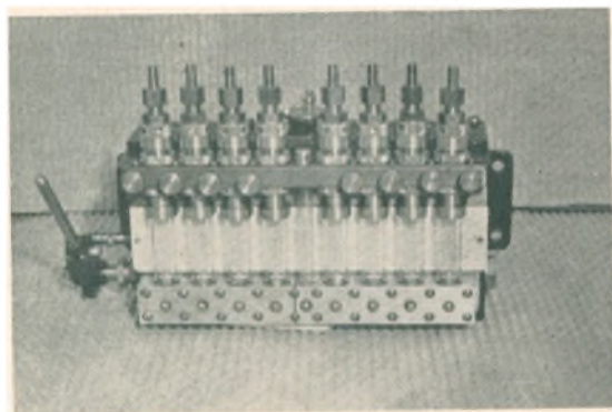
Smøreapparat
