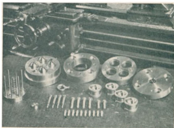
Form til Plasticstøbning
