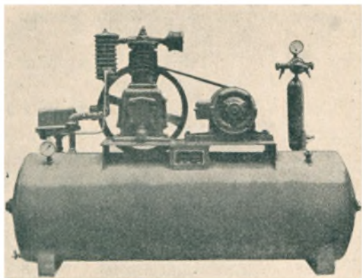
D.S.T. Kompressor
