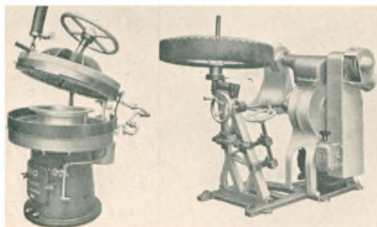
Top- og Helgummieringsform
