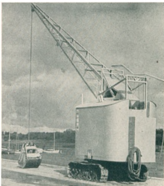
»H.N.« Kran leveret til Saxkøbing Havn
