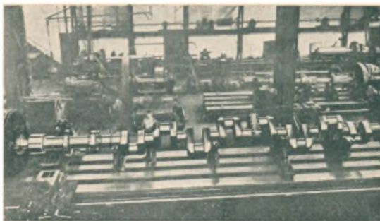
8-Slags Krumtapaksel med Trykaksel, Vægt 15 Tons Gussstahlwerk Witten
