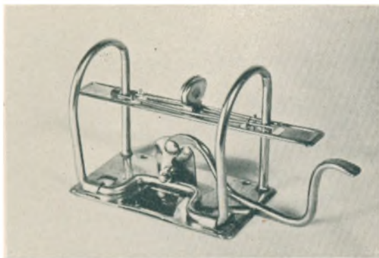
Lukkemechanisme til Brevordnere
