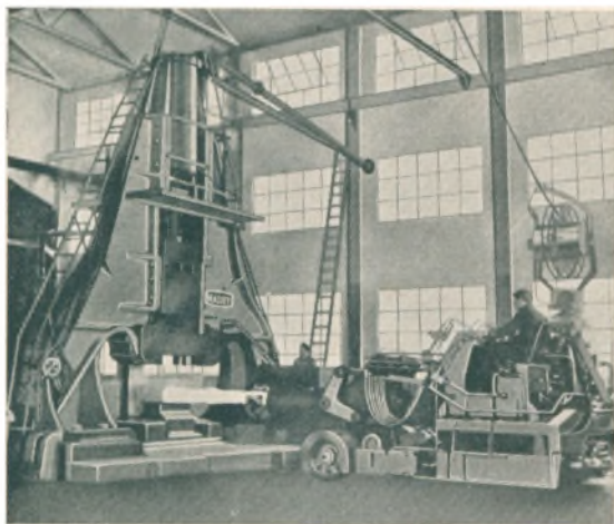
En af Hamrene ved Stavanger Electro-Staalverk
