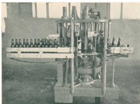
Etiketteringsmaskine
