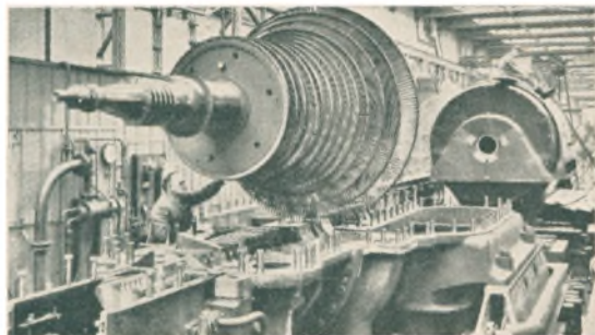
Indbygning af Rotoren i en Damp turbine , Maschinenfabrik Oerlikon, Oerlikon — Zürich
