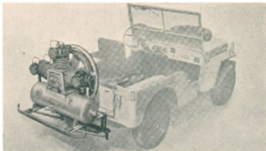
Kompressor paa Jeep
