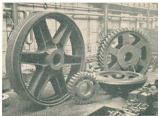
Svære Tandhjul (Gussstahlwerk Gelsenkirchen)
