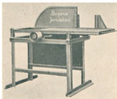
Moderne Rundsav
