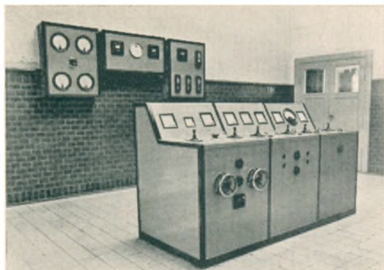
Pult- og Tavleanlæg for Elektricitetsværker i Virksomheden under Ledelse af Ingeniør Hans M. Falkenberg. Et Firma i rivende Udvikling.
