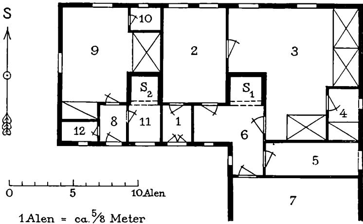
Grundplan af Stuelængen i den af Mads Chr. Jensen i 1846—48 byggede Gaard i Østtarp.
