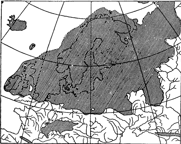
Fig. 1. Isens Udbredelse under den første store Istid (efter De Geer; her efter Salmonsens Konversationsleksikon).
