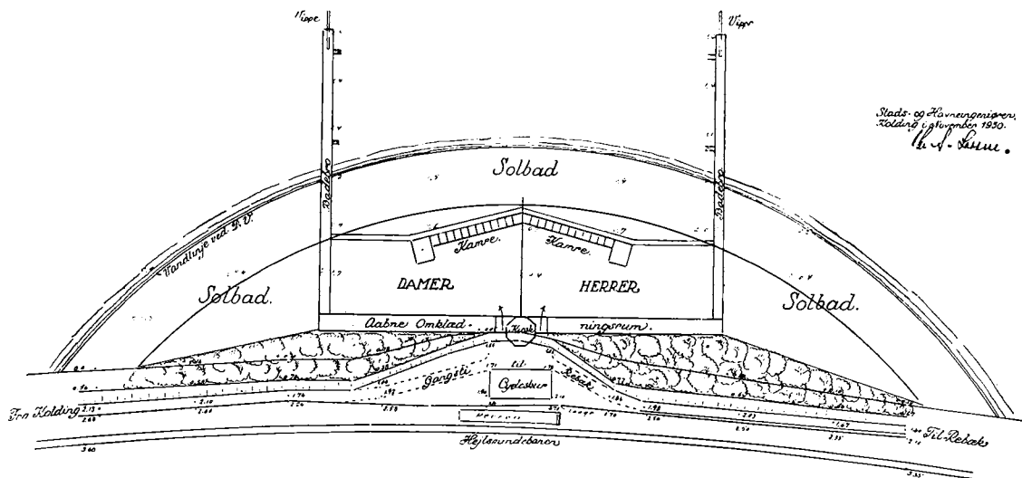
Det i Byrådsmødet Mandag den 17. November 1930 fremsatte Forslag til Ombygning af den komm. Søbadeanstalt.
