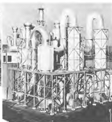
Anlæg til tørring af cellulose leveret af ingeniørfirmaet Niro Atomizer, Søborg, også medlem af DDS-gruppen.
