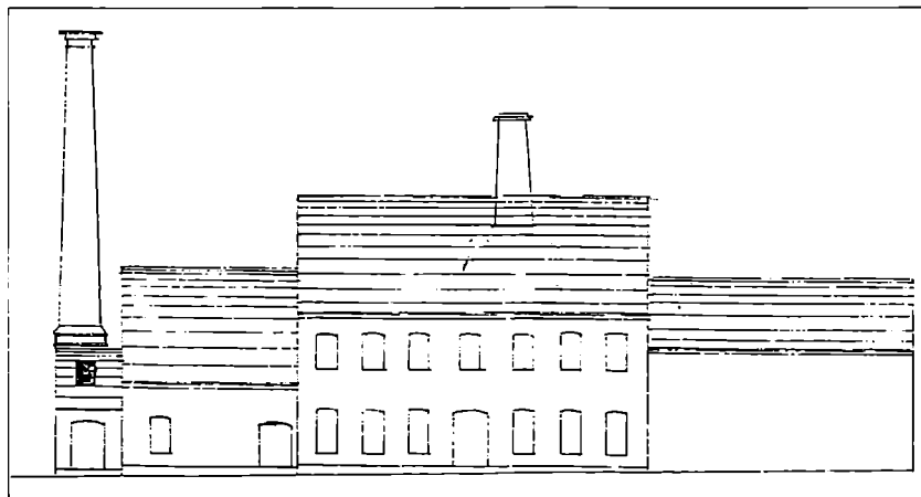
Snit af A.P. Jürgensens klædefabrik i Borggade, 1872. Fra venstre kedel- og maskinhus, i midten fabriksbygningen, til højre farveriet. Landsarkivet i Aabenraa, Aabenraa landråd PB9.
