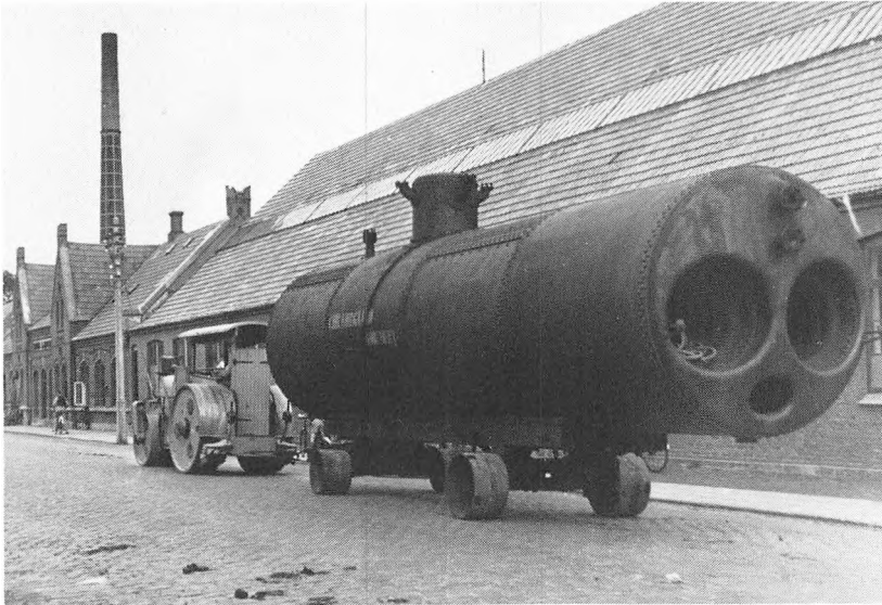
Den solide Lancashire kedel (100 m 2 hedeplade), der vejede 32 tons, måtte man have kommunens vejtrømler til at slæbe på plads.
