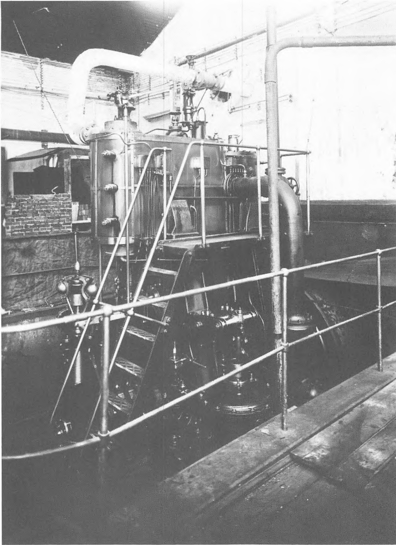
Dampmaskinen på 100 HK, der blev anskaffet i slutningen af 90'erne var en brugt skibsmaskine. Nu fik den sit otium i det indre af Jylland.
