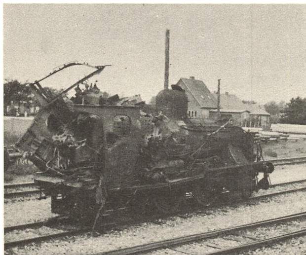
Det sønderskudte Lokomotiv paa Skærbæk Station.
