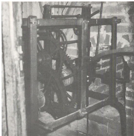
Tårnuret i Stenløse kirke. (N.M.)
