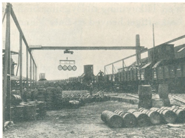
Phønix, Vejen: Vejmaterialefabrikens Krananlæg og Læsseanordning.
