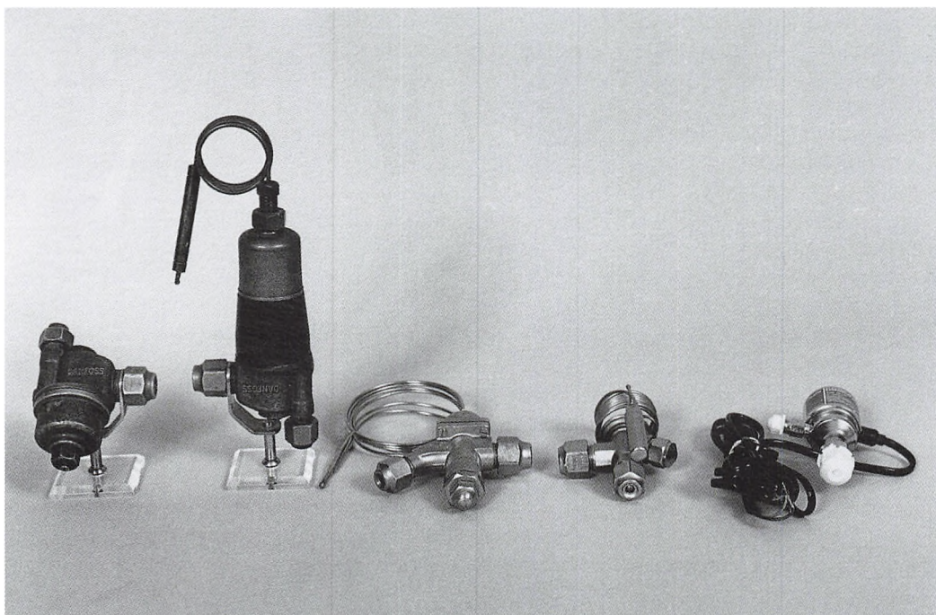
Billedet viser 60 års udvikling af Danfoss ekspansionsventiler til mindre køleanlæg. Yderst til venstre ses den automatiske (trykstyrede) ekspansionsventil, type ARV fra 1933 - samme år som Danfoss blev grundlagt. Få måneder senere fulgte den termostatiske (temperaturstyrede) ekspansionsventil, type TRV (nr. 2 fra venstre). De tre følgende produkter viser udviklingen af ekspansionsventiler frem til 1988.
