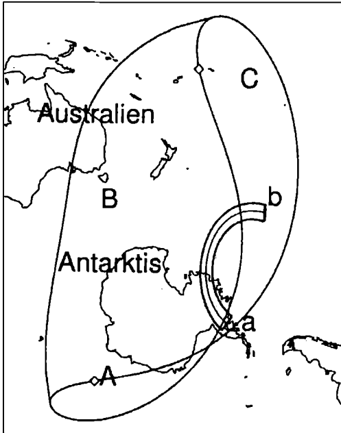
Ringformet solformørkelse 7. februar 2008
