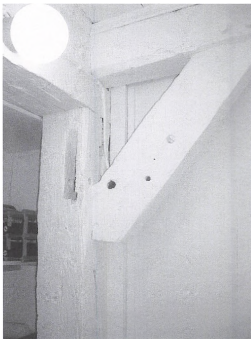
Højremskonstruktionen. Indvendig rem i spisekammeret i nordsiden med stolpe og kopbåndforbindelse til loftsbjælke
