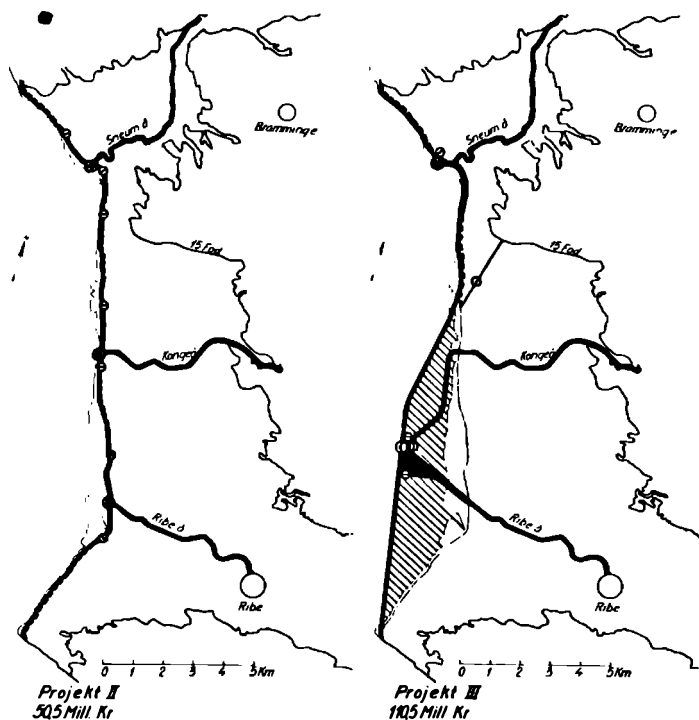
Fig. 14. 2 af de 5 alternative projekter, der i 1960 udarbejdedes til sikring af Ribbe-diget af det af Ribe amtsråd nedsatte teknikerudvalg.
