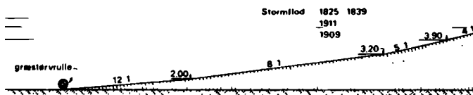
Fig. 13. Tværprofil af Ribe-diget fra 1912-24.
