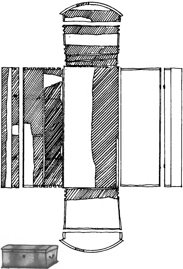
Fig. 7. Karnlågskiste. Tegnet fra udvendig side af bund i målestoksforhold 1:20. På opmålingstidspunktet var det skraverede bevaret. H81.
