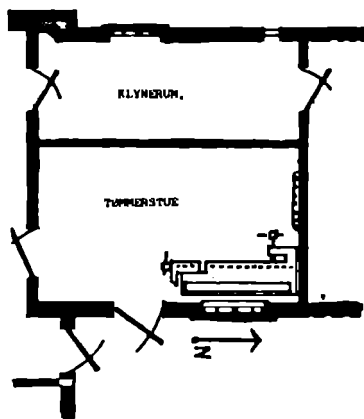
Fig. 3. Hougård 1863-1928. Det skraverede er Tømmerstuen. Målestoksforhold 1:400. H81.
