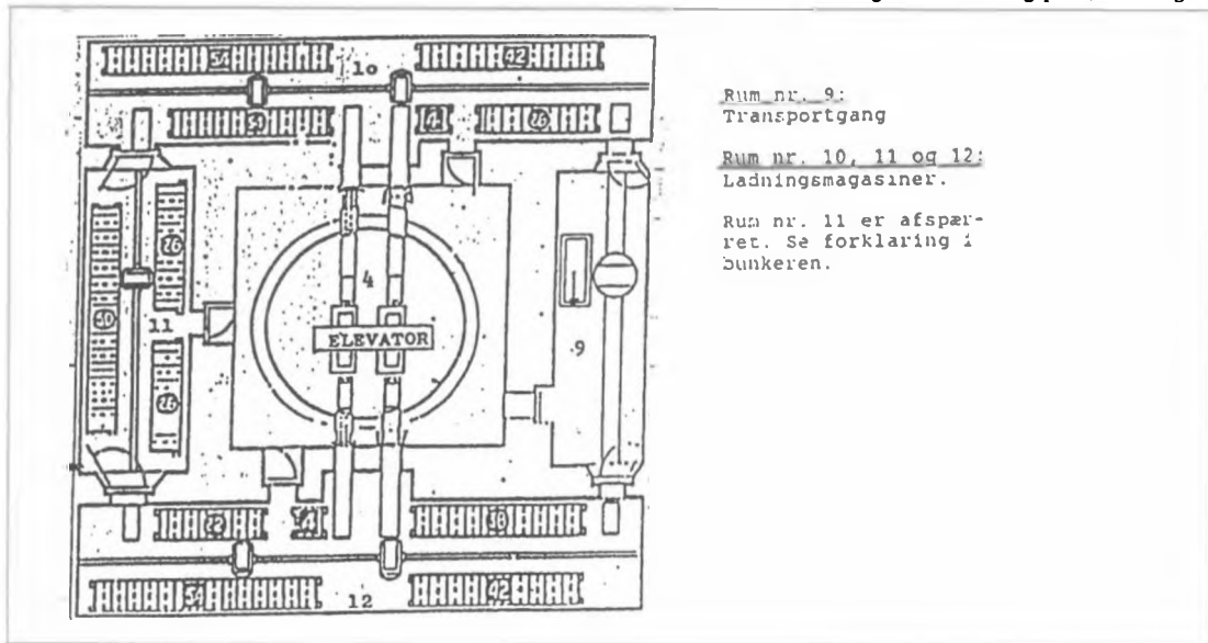
Fig. 10. Indretningsplan, overetagen.
