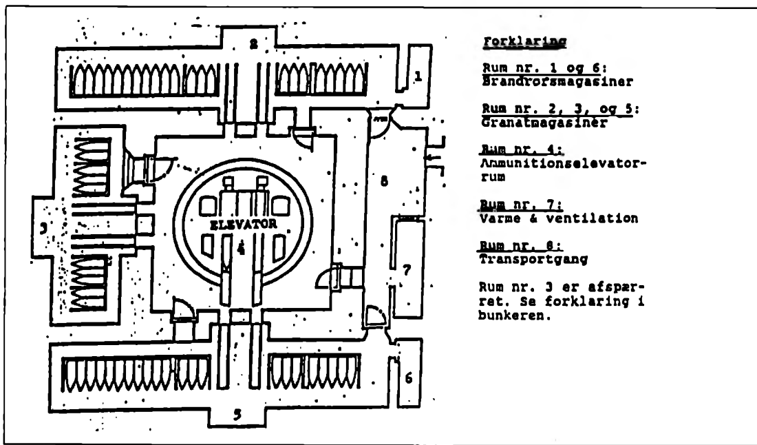
Fig. 9. Indretningsplan, underetagen.
