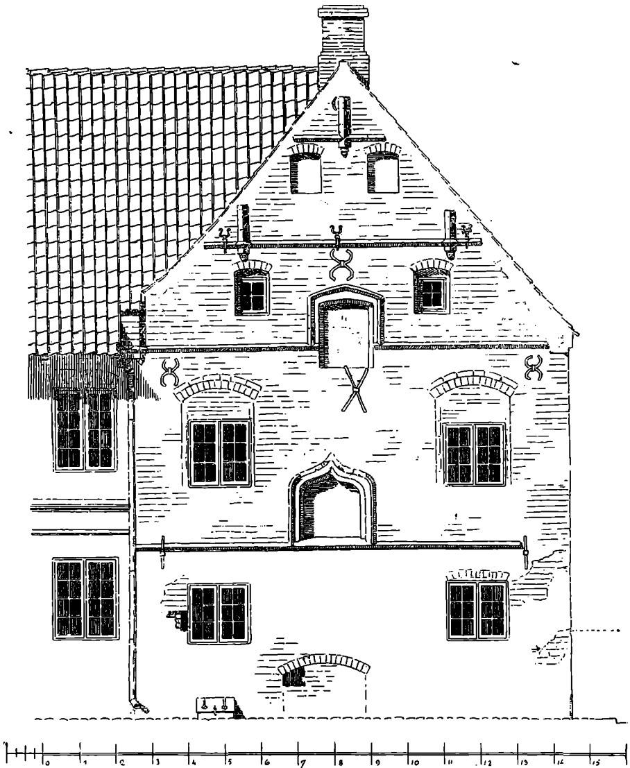
Vestgavl af Sydføljen. Opmaalt for Nationalmuseet af Holger Hagemann.
