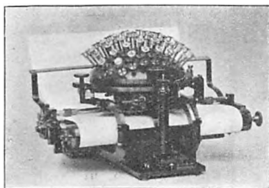
Den allersidste Model af Malling Hansens Skrivemaskine, den saakaldte Vippe-kugle, der fungerer uden elektrisk Tilbehør.
