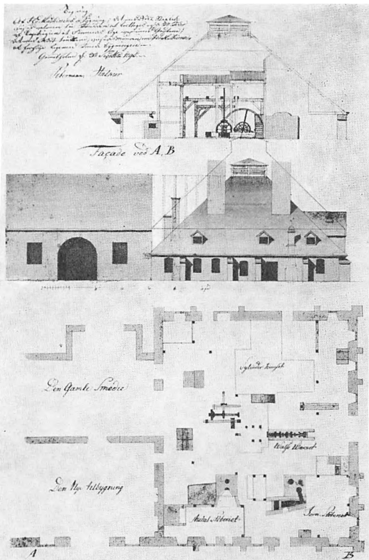
Ildmaskinhuset på Bremerholm, i hvilket Danmarks første dampmaskine blev anbragt. Her er de approberede tegninger, udført af murermester Petermann og tømrermester Halkier.
