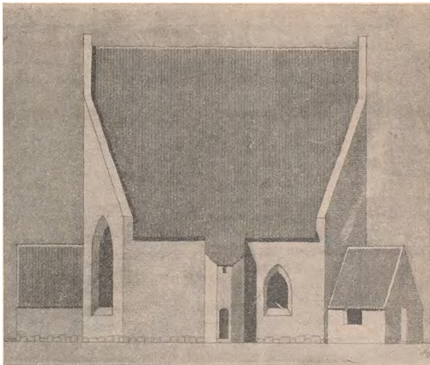
Projekt til kirke i Brejning, tegnet i 1941 af professor Mogens Kock, opført 1966. Foto: Mogens Kock.
