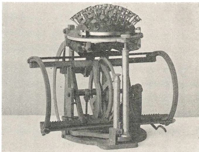
Skrivekuglen, Forløberen for den nuværende Skrivemaskine, opfundet af Danskeren Malling Hansen.
