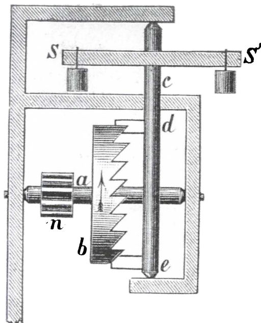
Nok var spindelgangen en enkel konstruktion, men for de tidligste urmagere voldte det store problemer at fremstille f.eks. kronhjulets stærkt tilspidsede, underskårne tænder. Ill. Bering-Liisberg: Urets Udvikling. København, 1905.
