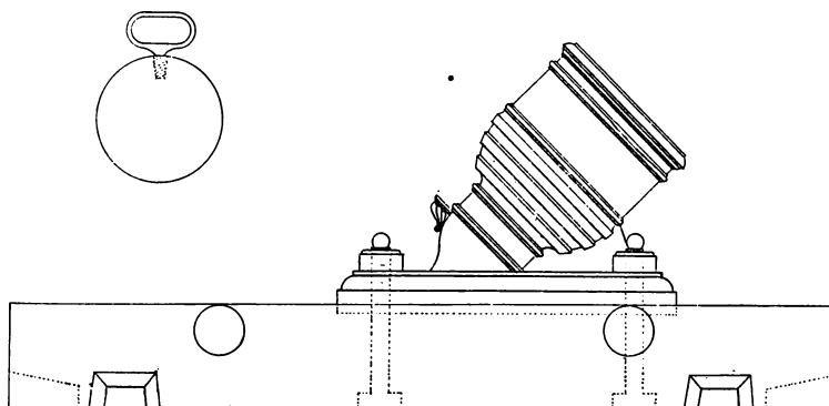
SIDE AF EN BOG MED TEGNINGER OG MAAL AF FREDERIKSVÆRKSKE KANONER M. M. Tegnet af Boremester S: Juncker.
