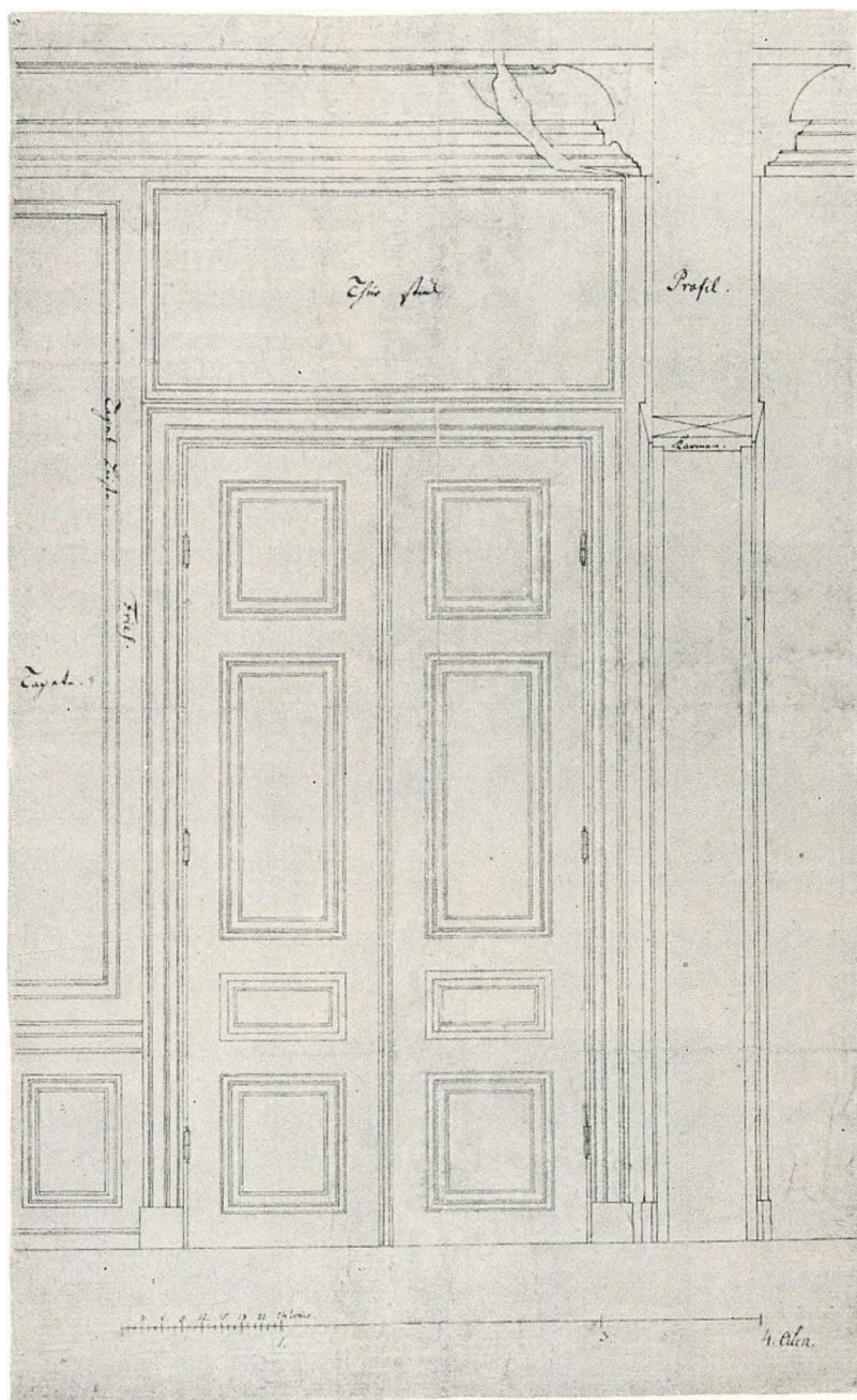
Langesø. Tegning til Flojddør. Formentlig fra Opførelsestiden.
