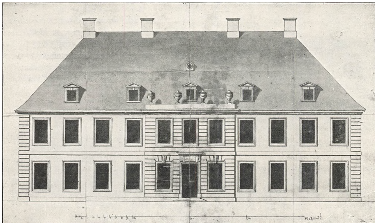
Langsø. Projekteret Façade, sandsynligvis mod Haven, tegnet af J. E. Rosenberg I Hovedtrækkene svarer denne Tegning til Bygningens nuværende Udseende Bag paa Tegningen findes følgende Paaskrift: Forevist ved Forretningen paa Langsø d. 6te Jan. 1776
