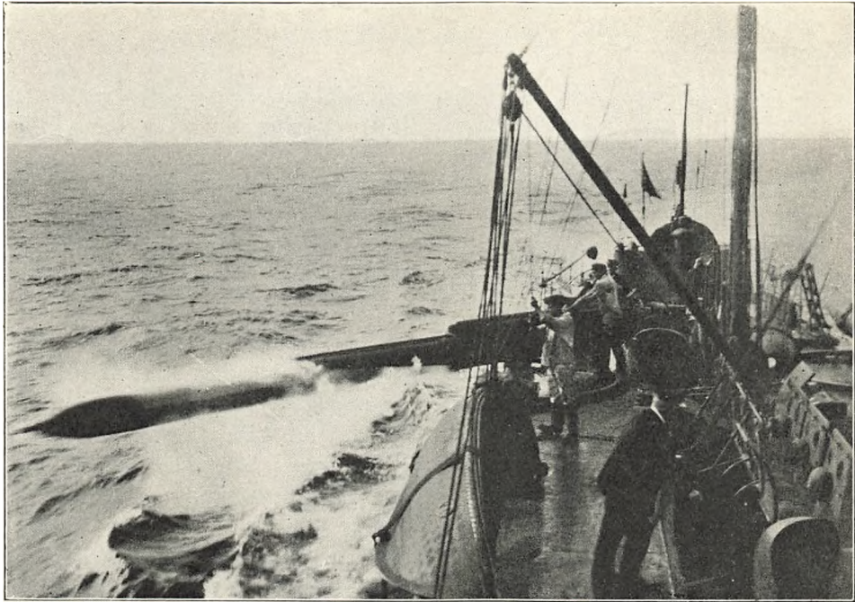
Torpedoskud fra Dæksapparat.
