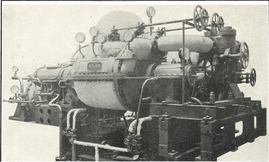
3000 HK. gearret Atlas-Turbine til »Dragen« — Baad.
