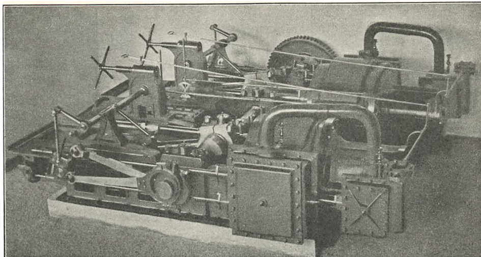
552 HK. Tandem-H. og L.T.-Maskine. Krydserskorvetten »Fylla« 1852.
