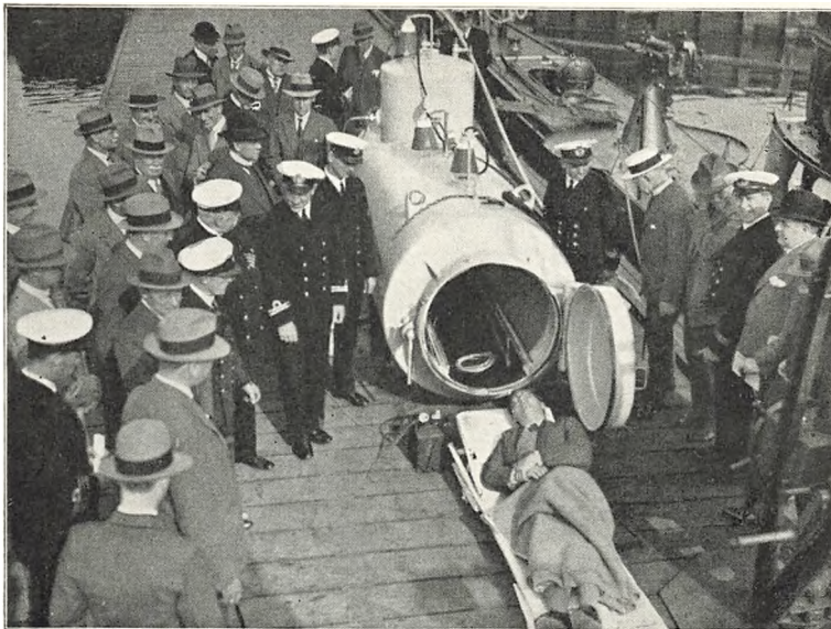
Dekompressionskammeret demonstreres.
