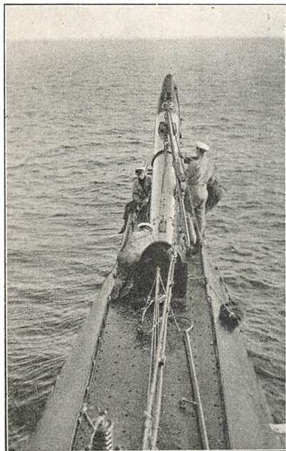
Torpedoen føres ned »om Læ« efter Skud.
