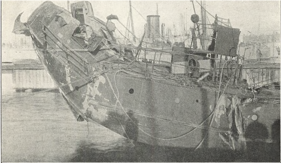
»Sværdfisken« Agterende efter Minesprængningen.
