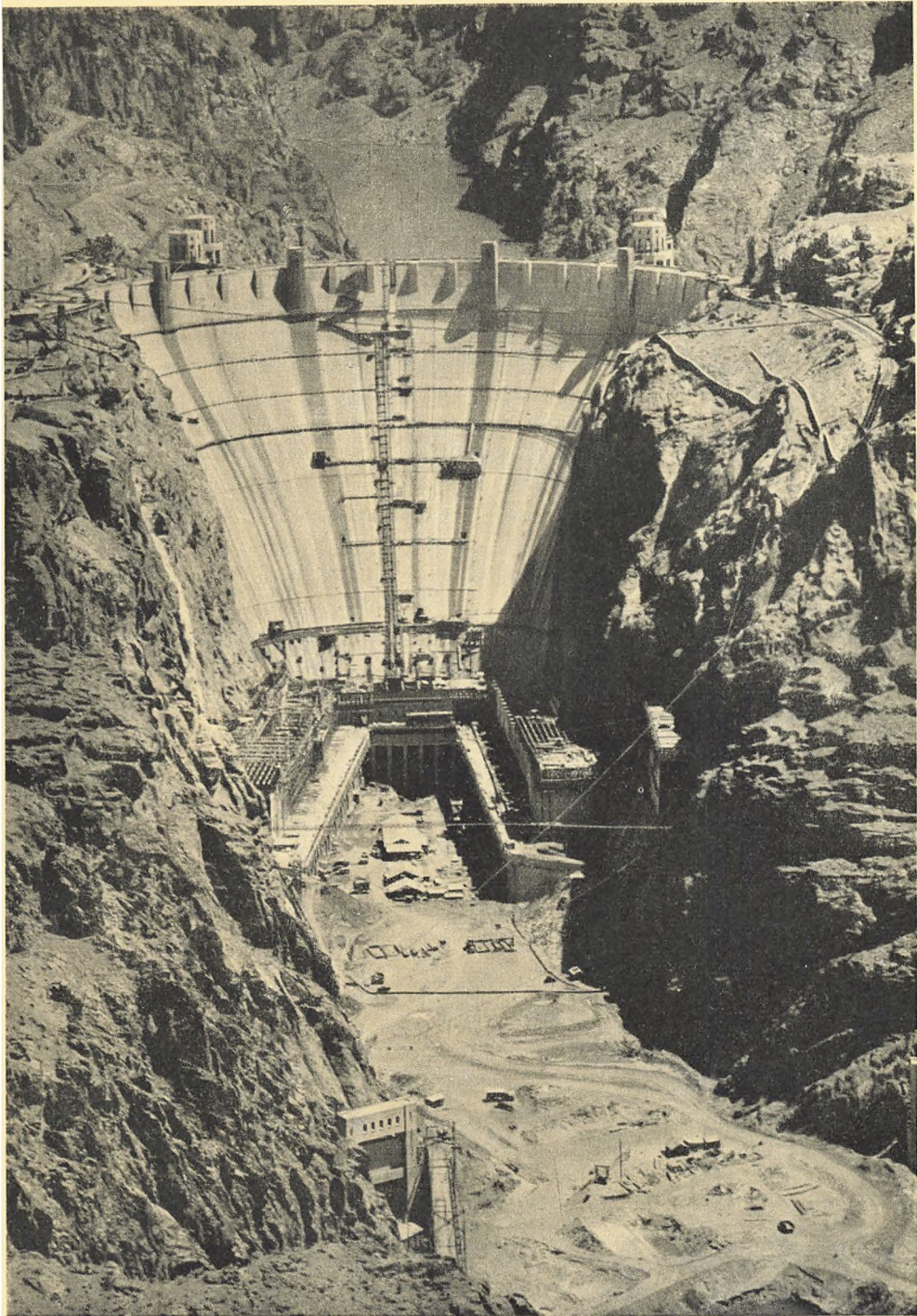
Boulder Dam, i hvis Projektion Danskerne Ingeniør Lars Jørgensen og Professor H. M. Westergaard har deltaget
