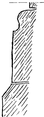
Den dobbelte profile- rede Sokkel under Kirken.
