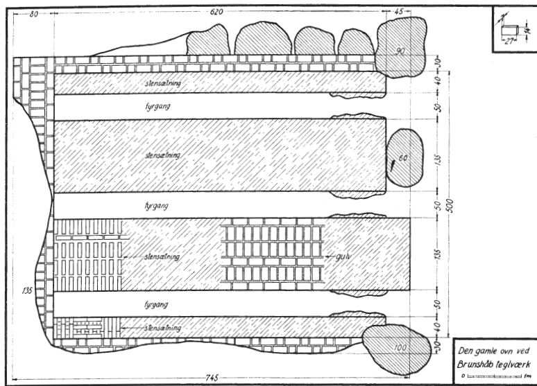
Fig. 16. Tegllovn fra Bruunshaab undersøgt i 1938. Tegning: B. Gulddal (fra M.E. Gulddal: En middelalderlig tegllovn fra Bruunshaab, i: Fra Viborg Amt, 1958, s. 11 ).
