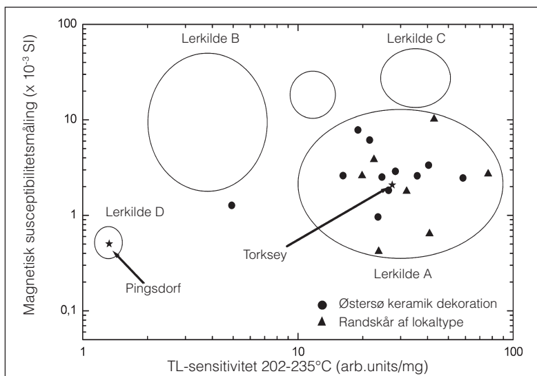
Fig. 14. Magnetisk susceptibilitetsmåling på randskær af lokaltype, keramik med Østersøkeramikdekoration, engelsk Torkseydekoration og et tysk importskær fra Pingsdorf i Rhinområdet. Alle skårene stammer fra Sønderløområdet.
