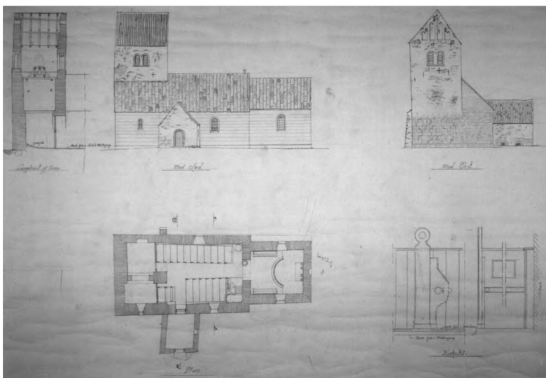
Vester Tostrup Kirke før ombygningen i 1928, opmålt af arkitekt Søren Vig-Nielsen. Man bemærker tårnets skæve placering og dets fundament i skibets fulde bredde. Udvendig mod nord er vist støttepillen i overgangen mellem tårn og skib. Inde i kirken ses den svære midterpille og den murede adskillelse mellem skib og tårn på begge sider af denne. Endvidere ses mod syd det ligeledes oprindelige, skæve våbenhus. I tårnets nordsokkel samt i begge sokkelsider på våbenhuset ses de indmurede romanske vinduesoverliggerere.
