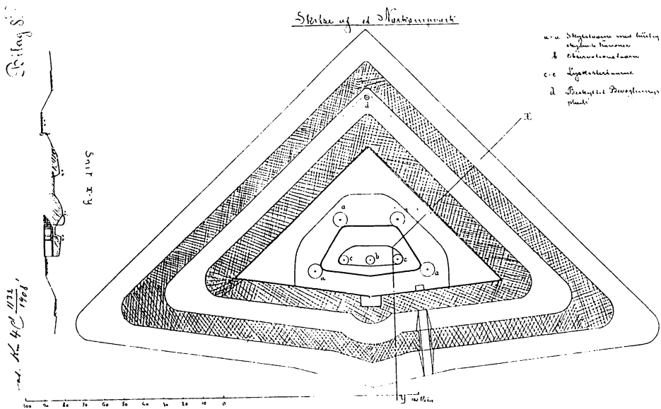
Skitse til et af de 'fremskudte forter'; et af de egentlige befæstningsanlæg, der skulle understøtte den fremskudte feltbefæstning. I det projekt, der blev skitseret i skrivelsen af 30/11 indgik der 11 forter, 10 maskingeværzanlæg og 52 batterier med i alt 244 stk. artilleri og 670 maskingeværer; alt i alt ikke noget ubetydeligt befæstningsanlæg.
