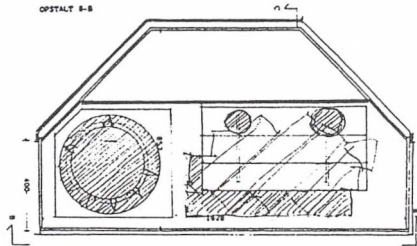
PLANSNIT A-A
