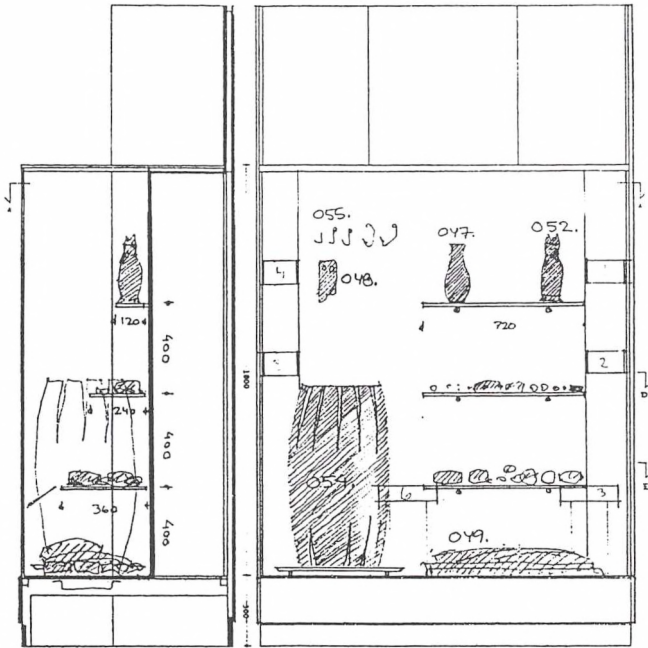
LØSRET SNIT C-C
