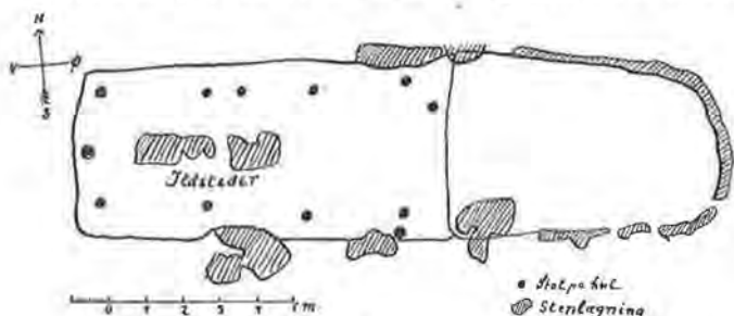
Grundplan af det største Tolstrup-Hus.
