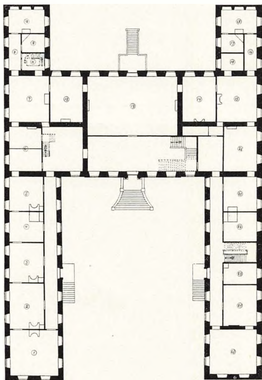
CLAUSHOLM. PLAN AF STUEN.
