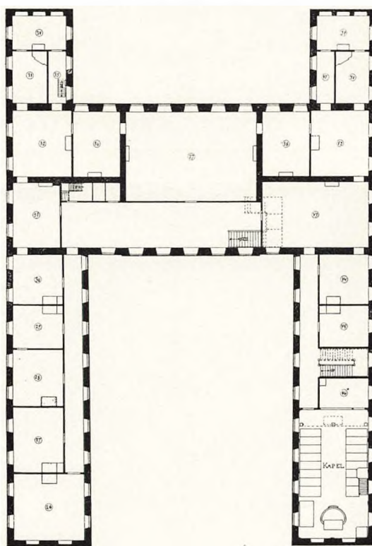
CLAUSHOLM. PLAN AF 1 STE SAL.
