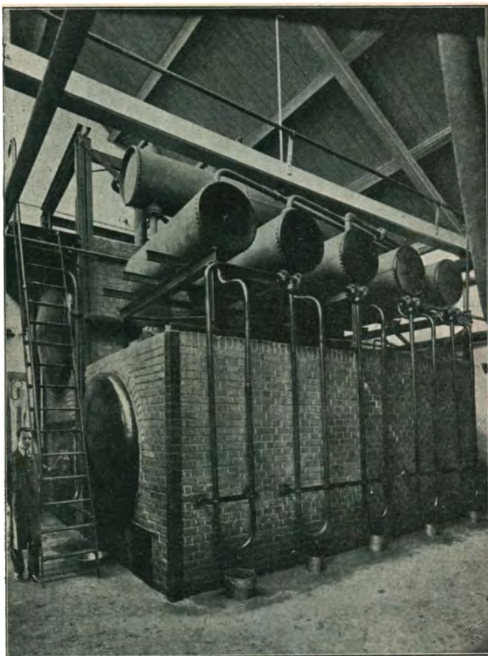
Destillationskedel med Forvarmer og Deflegmatorer 1901.
