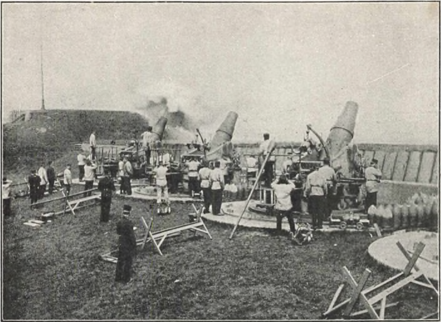
28,5 cm Haubitsbatteri i Virksomhed paa Lynetten.
