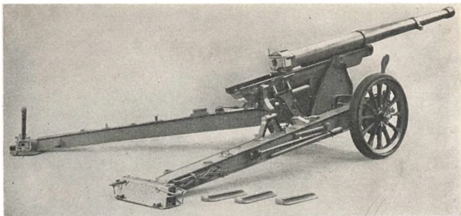
10,5 cm Feltkanon, Model 1930.
